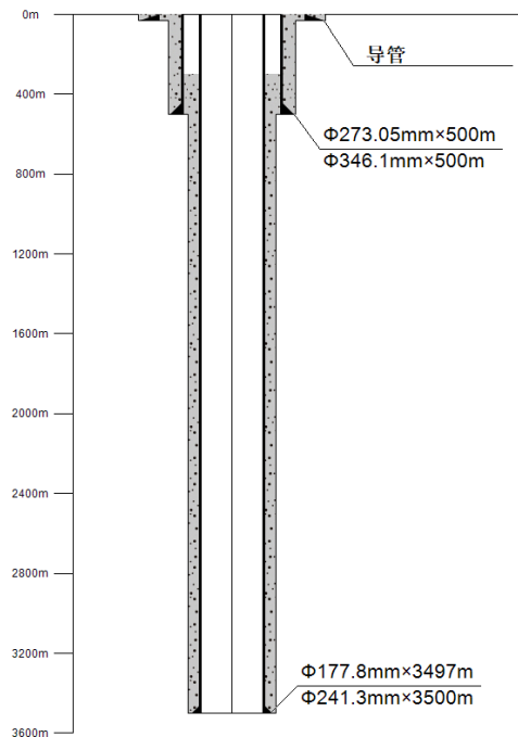
图 2-3 直井井身结构示意图
