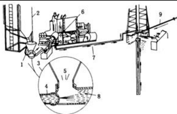
1-下类漏斗：2-供灰罐：4-水的喷射：5-快速下灰：6-固井泵吸灰浆： 7-向套管内注入泥浆：8-水和水泥混合成水泥浆情况：9-钻井液循环管线
