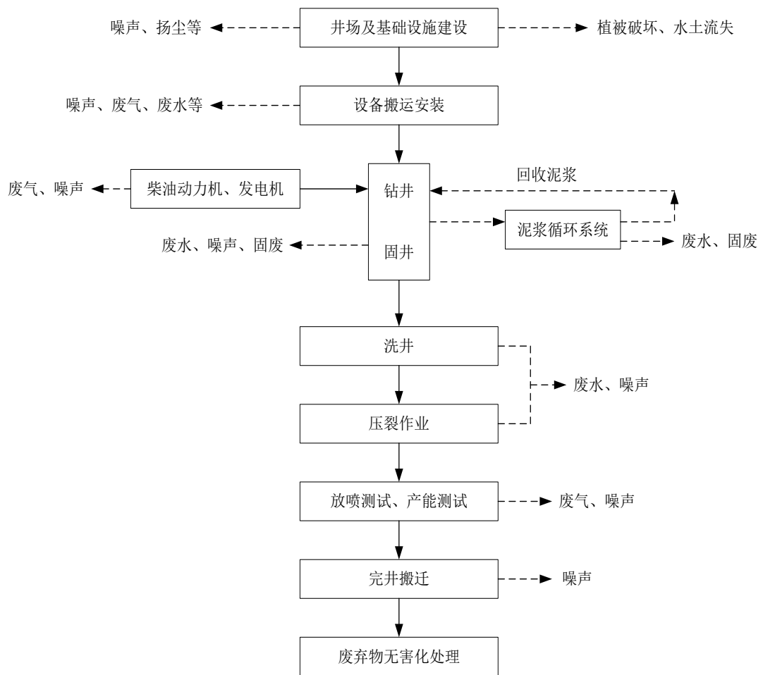
图 2-2 钻井工艺流程图及产排污节点示意图
