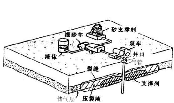
图 2-6 压裂作业示意图
